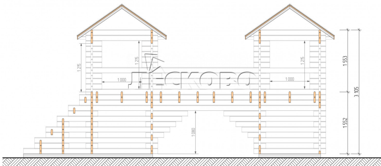
Разрез
