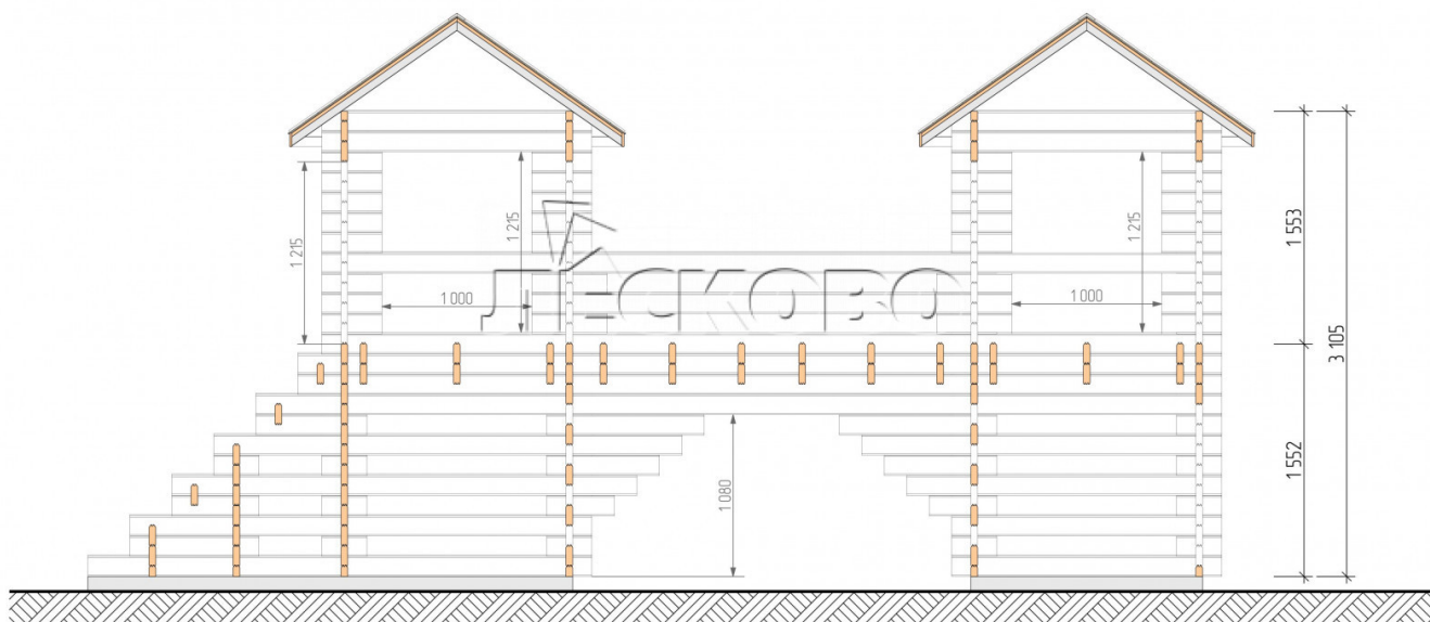
Разрез
